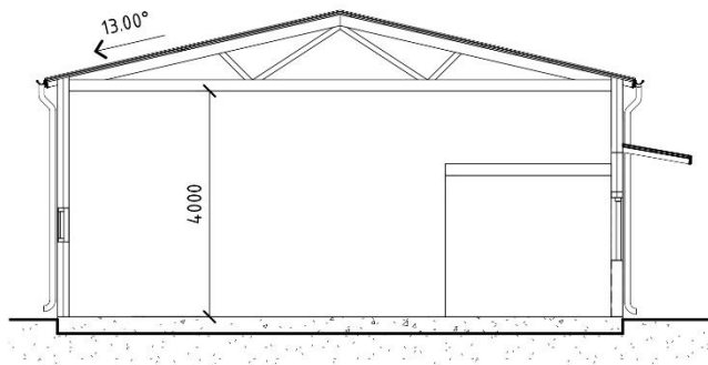
SEKTION A-A
